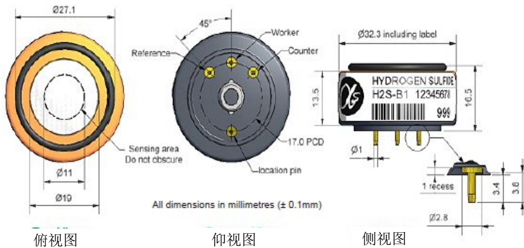
图1 H2S-B1示意图
