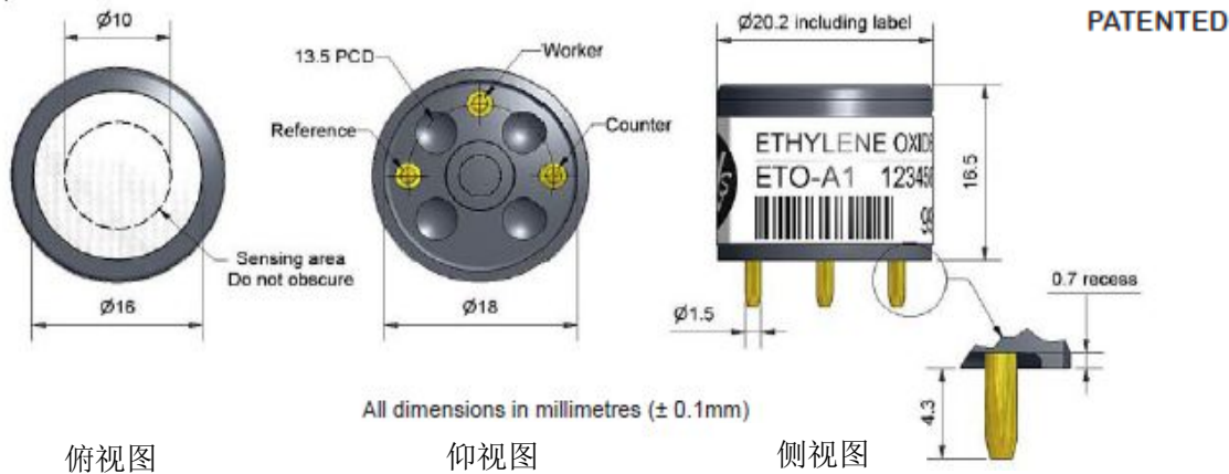
图1 ETO-A1 示意图
